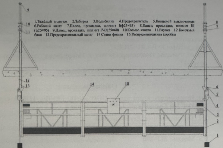
Рис. 1. Фасад электрической подвесной люльки
