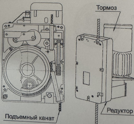
Рисунок 4 – Приводная лебедка
