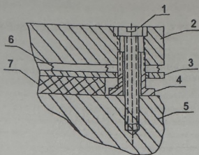
Рисунок 14 – Электромагнитный тормоз
