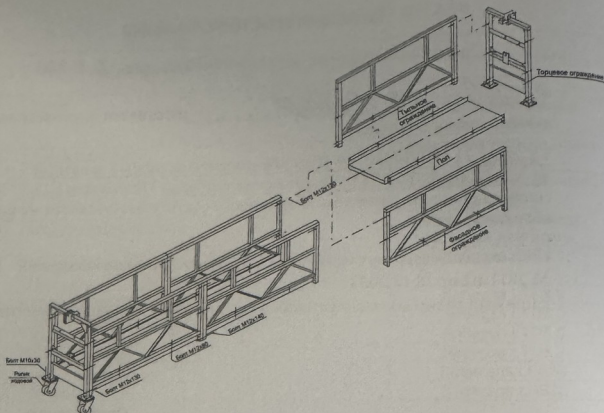
Рисунок 3 – Сборка люльки фасадного подъемника
