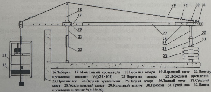
Рис. 2. Профиль электрической подвесной люльки
