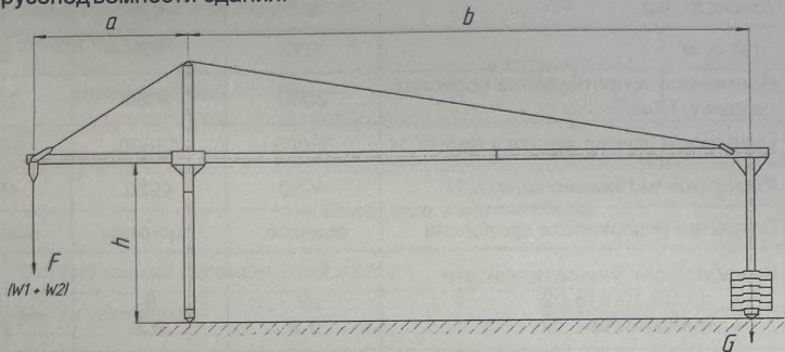
Рис. Схема для расчета устойчивости устройства для подвешивания платформы
