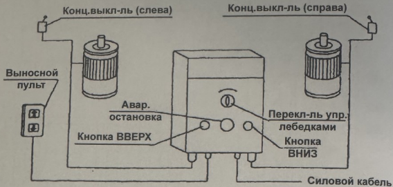
Рисунок 12 – Пульт управления подъемником
