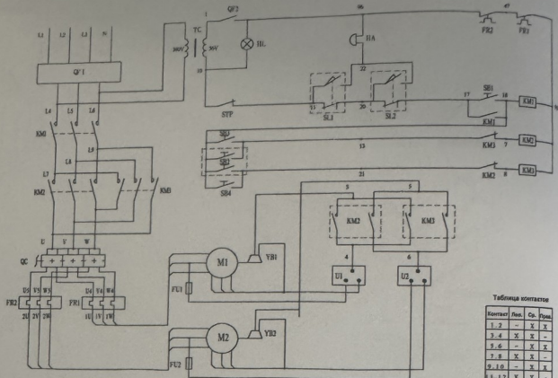
Рисунок 10 – Схема электрическая принципиальная
