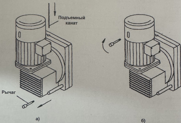
Рисунок 13 – Устройство ручного растормаживания
