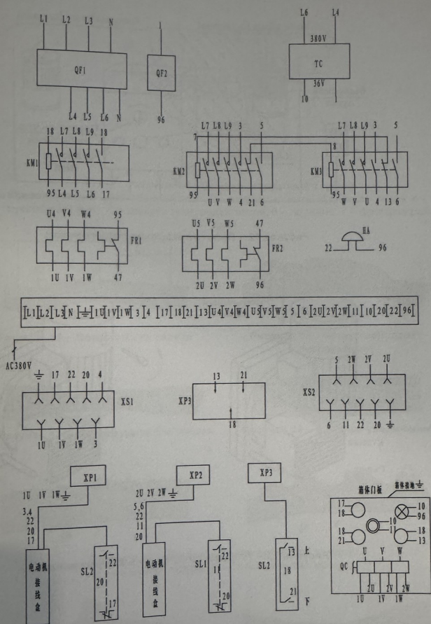
Рисунок 11 – Схема электрических соединений со спецификацией
