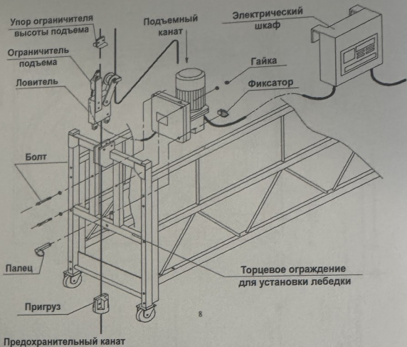
Рисунок 7 – Установка ловителя подъемника
